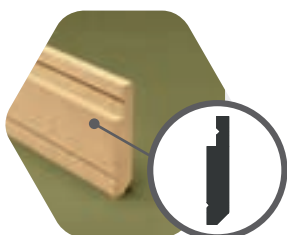
Installatiekit Lambris, bestaande uit sokkel 18 x 90 x 2400 mm 3 bevestigingslatjes 10 x 25 x 2400 mm 718135
