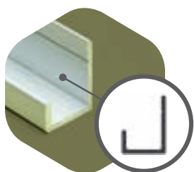
Eindprofiel ALU 7,4 x 13,4 x 18 x 2700 mm 500960
