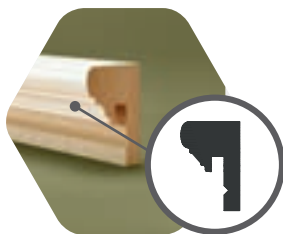
Profiel Lambris 38 x 57 x 2400 mm Classic (1 stuk per pak) 717856
