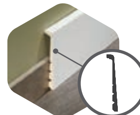
Universele overzetplint 16 x 130 x 2400 mm (2 stuks per pak) 717927
